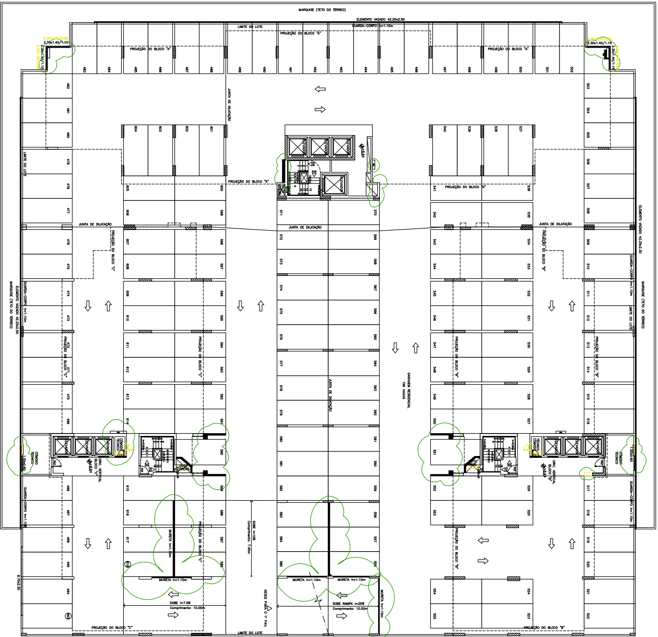
PLANTA - 2º PAVIMENTO ESCALA 1/100
